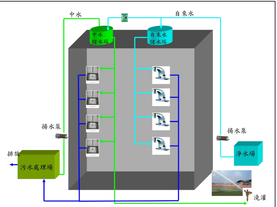
中水回收配置圖
