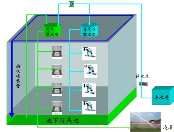
雨水回收配置圖
